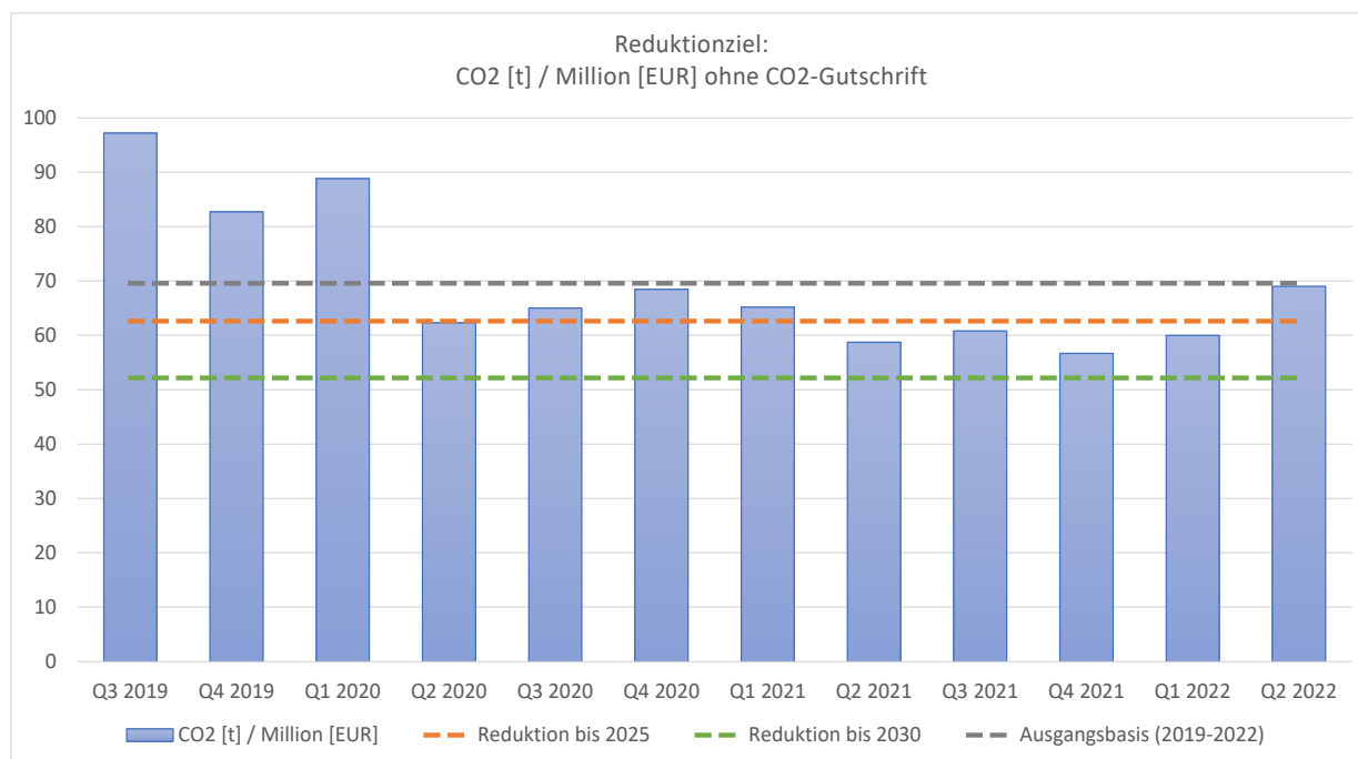
Abbildung 1: Reduktionsziele fair-finance
